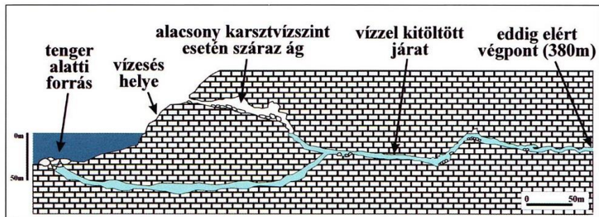
A Kotori-öbölben fakadó Sopot-forrás barlangjának hosszszelvénye (Stefanovic et al. 2010 alapján)
